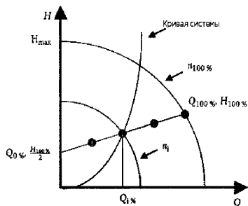
Рис. 2. Кривая системы интегрированного циркуляционного насоса.
